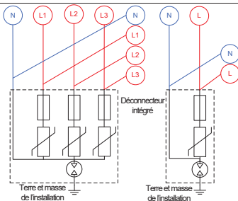
Schéma C2 : mode commun et mode différentiel
