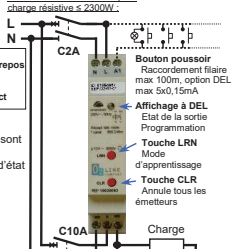
Schéma de raccordement pour charge résistive < 230W.
